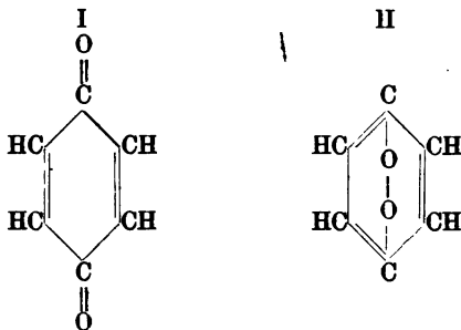
Chinon.
